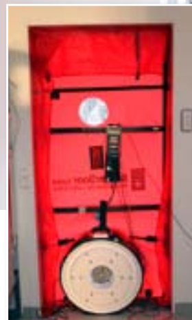
Provtryckningsaggregatet i ytterdörren.
