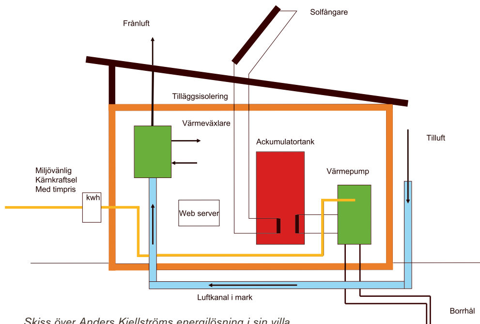
Skiss över Anders Kjellströms energilösning i sin villa.
